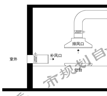
图 7.5.4 厨房补风示意图
