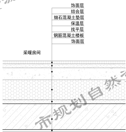
图 7.1.5-1 非采暖地下室顶板保温构造示意图 1
